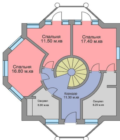
План второго этажа
